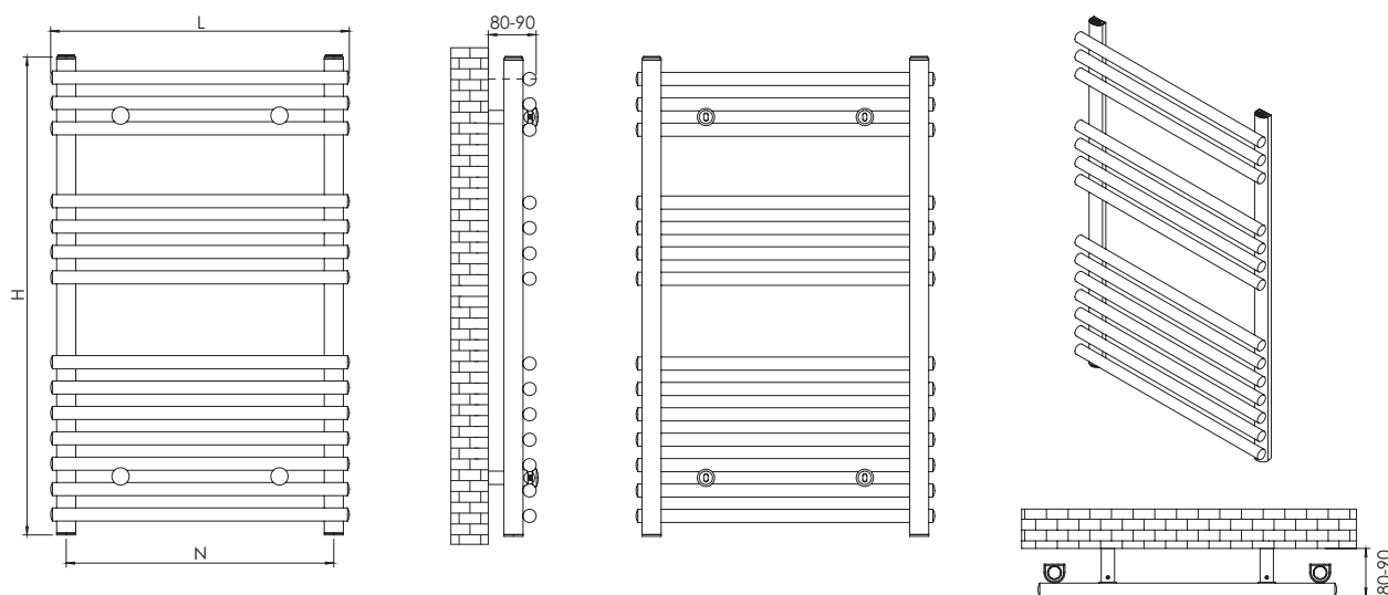
14/20/31 Tubi/Tubes
