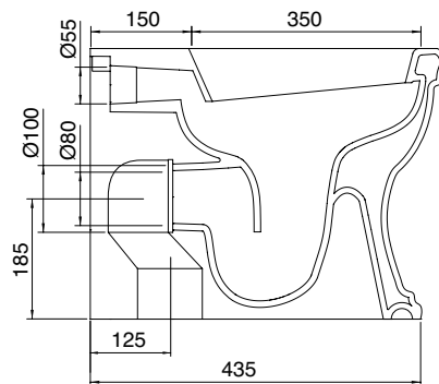
SEZIONE A-A
